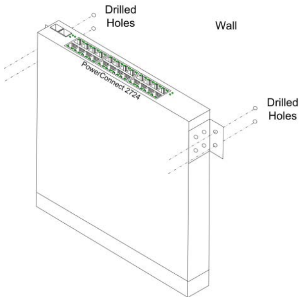
Figura 3-4. Montaje del dispositivo en una pared
