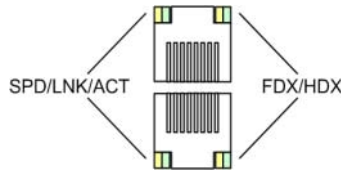
Figura 2-9. LED de RJ-45 10/100/1000BASE-T de cobre
