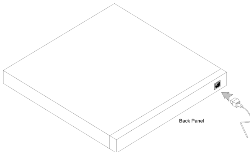
Figura 3-5. Conector de alimentación del panel posterior
