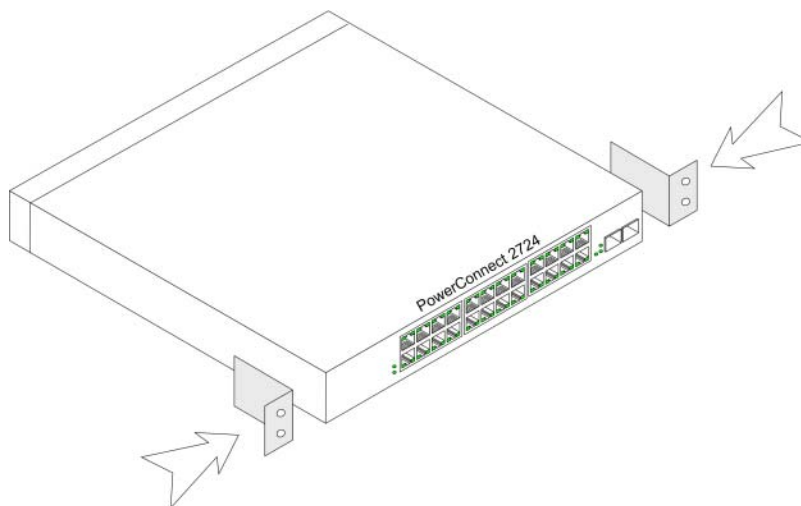
Figura 3-2. Montaje de los soportes para la instalación del rack
