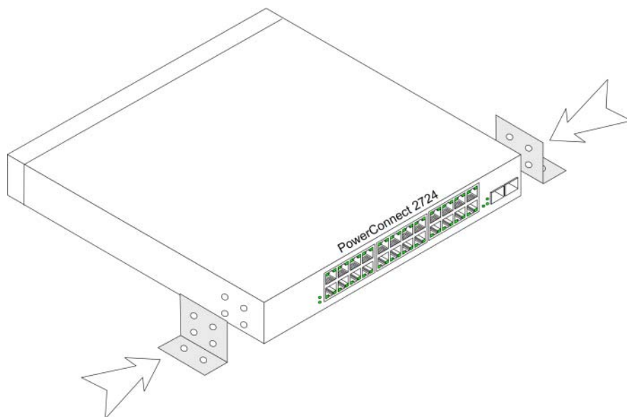
Figura 3-3. Instalación de los soportes para el montaje en pared
