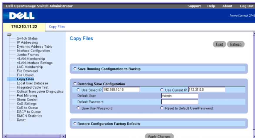
Figura 6-11. Copiar archivos
