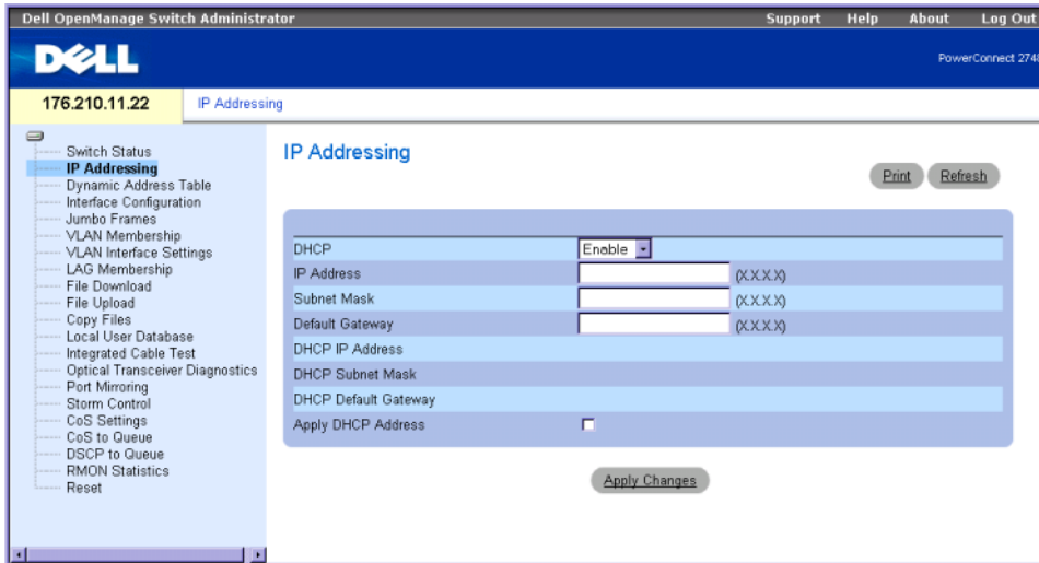
Figura 6-2. Direccionamiento IP
